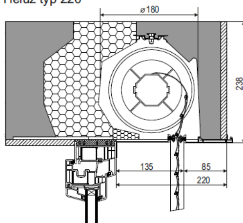
Heluz typ 220
