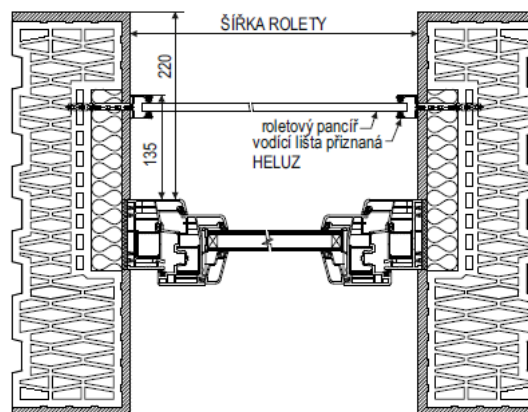
Heluz typ 220
