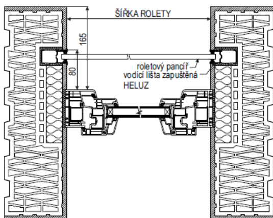
Heluz typ 165
