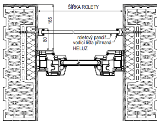
Heluz typ 165
