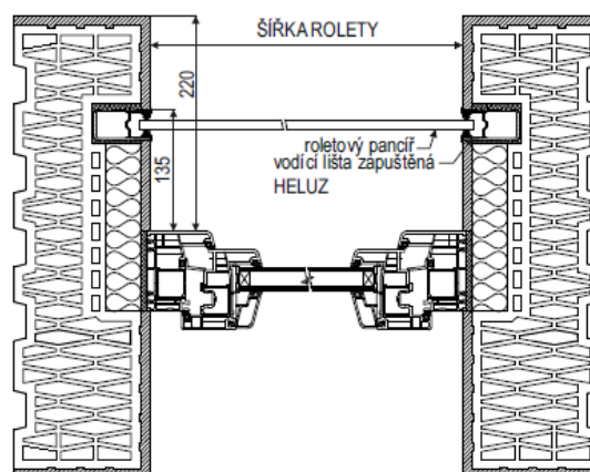
Heluz typ 220
