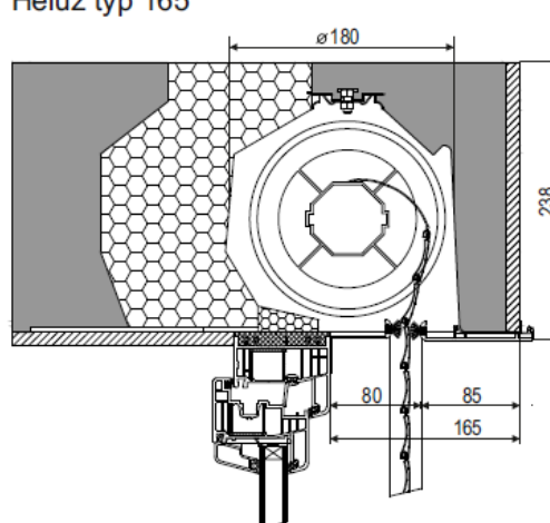
Heluz typ 165
